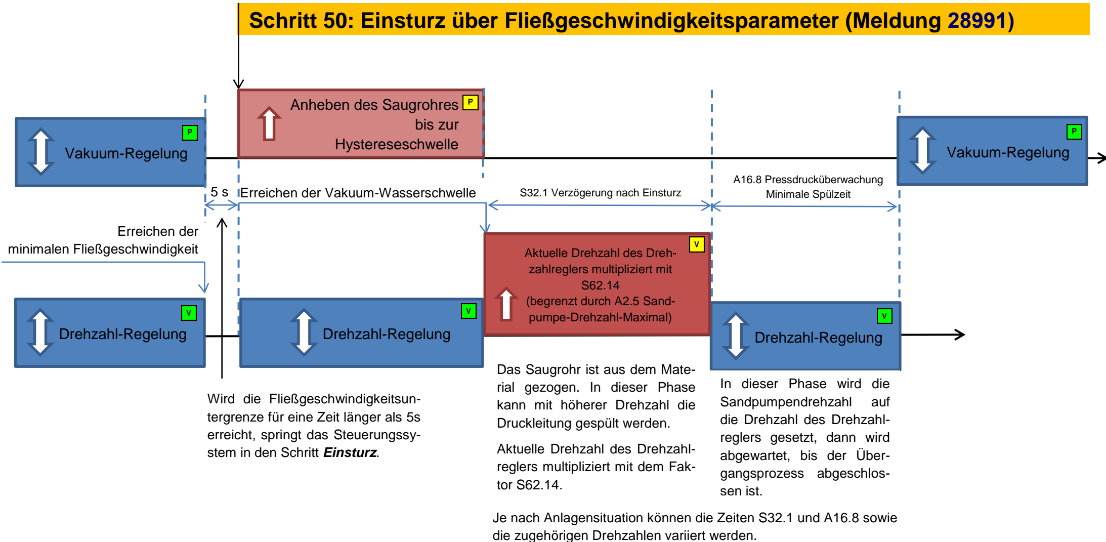
Timing-Diagramm beim Einsturz durch minimale Fließgeschwindigkeit S70.1
